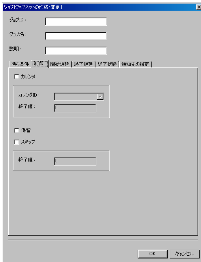
図 13-18 ジョブ[ジョブネットの作成・変更]ダイアログ (制御タブ)
