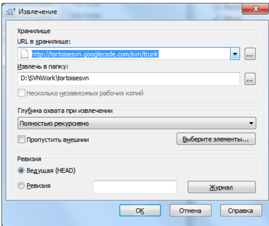
Рисунок 4.7. Диалог извлечения
