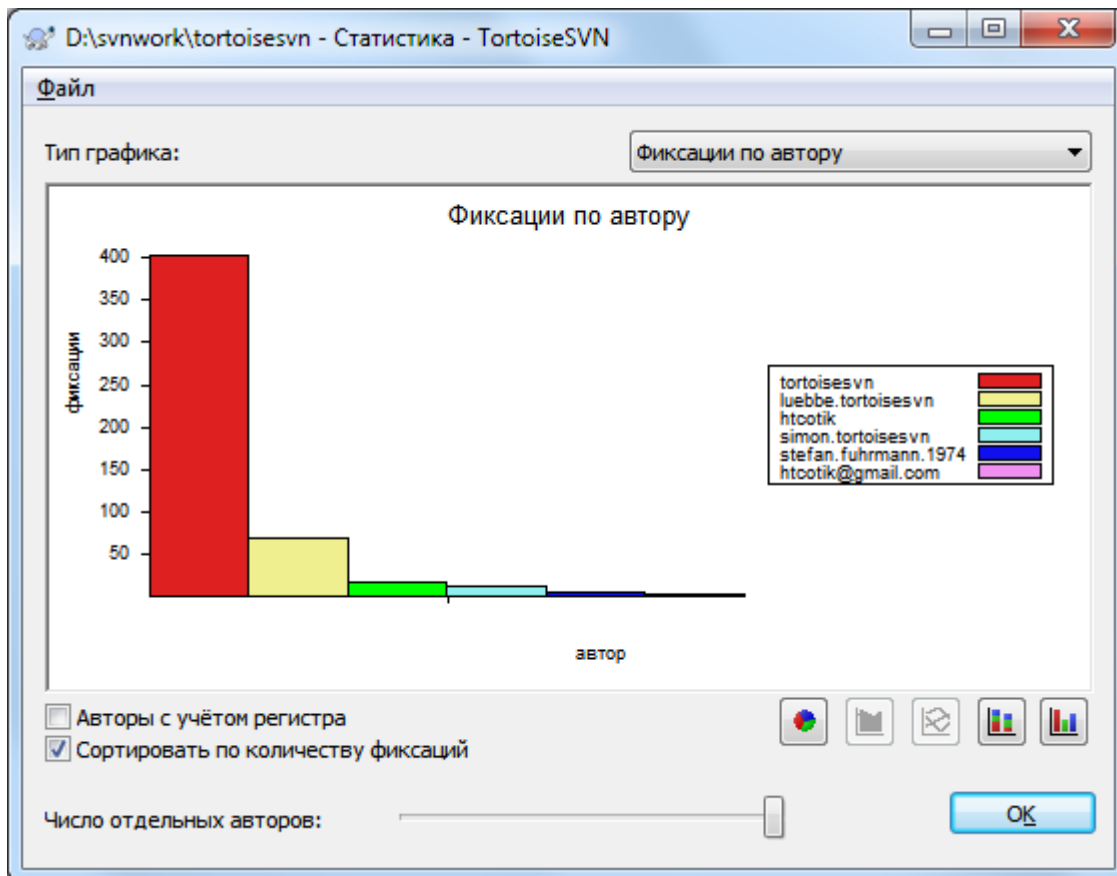
Рисунок 4.23. Гистограмма Фиксации-по-автору
