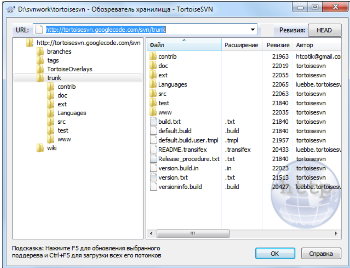
Рисунок 4.62. Обзорщик хранилища
