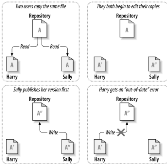
Рисунок 2.4. Модель Копирование-Изменение-Слияние
