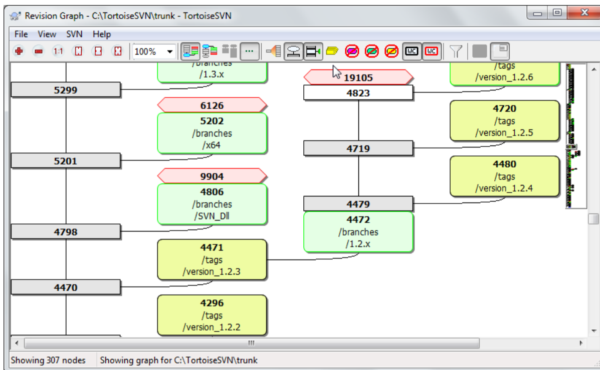
Slika 4.64. Graf revizije
