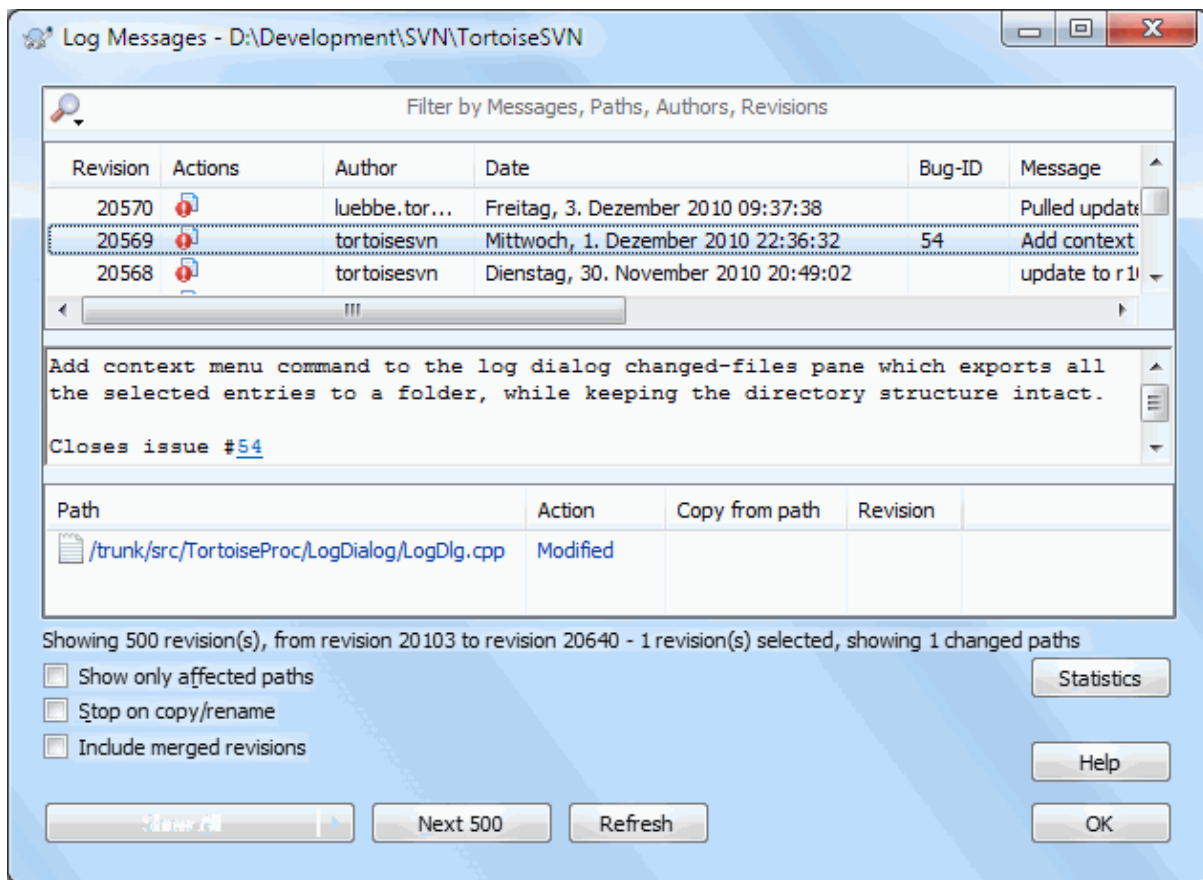
Slika 4.16. Okno dnevnik
