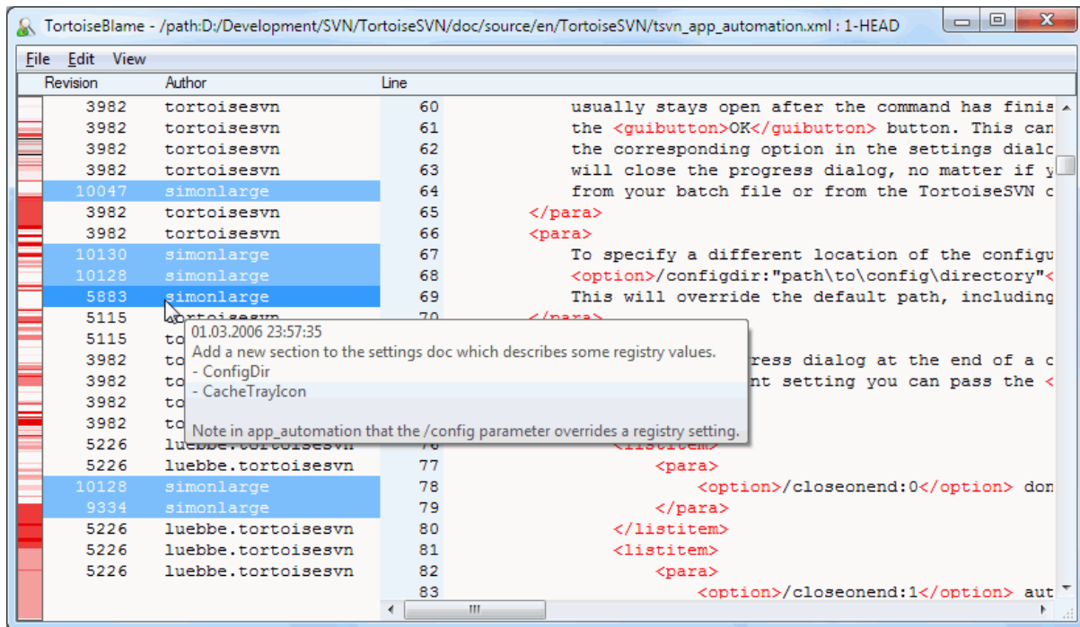
Slika 4.62. TortoiseBlame
