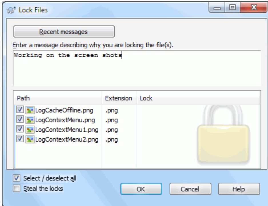
Obrázok 4.58. Dialóg zamykania
