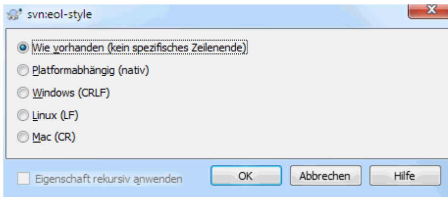
Abbildung 4.43. svn:eol-style Eigenschaftsseite
