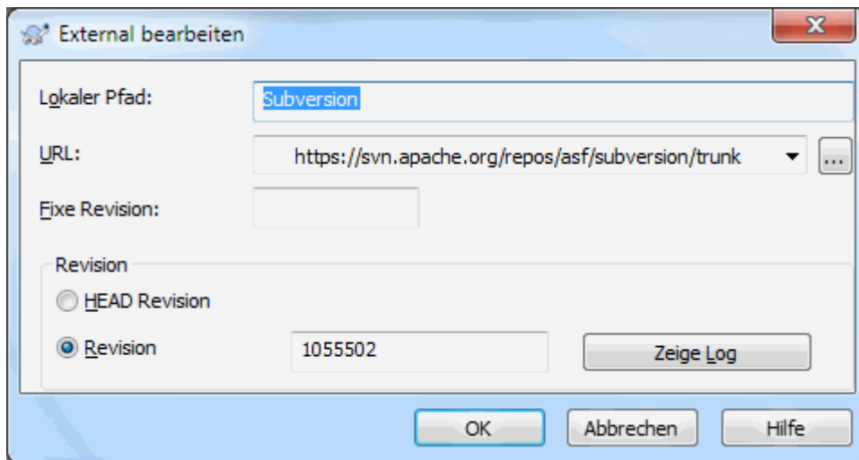
Abbildung 4.41. svn:externals Eigenschaftsseite
