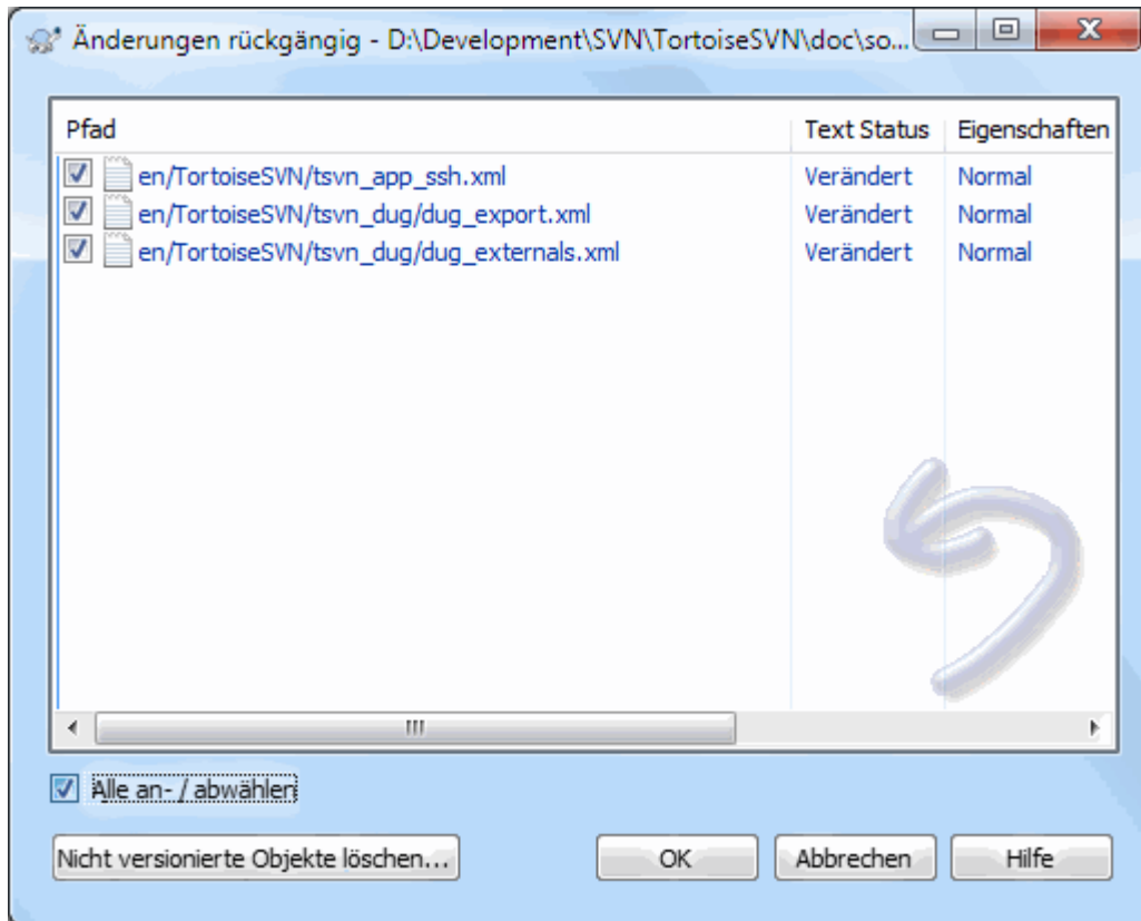
Abbildung 4.35. Rückgängig-Dialog
