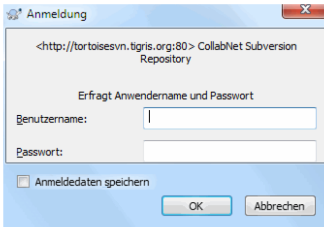
Abbildung 4.5. Anmeldedialog
