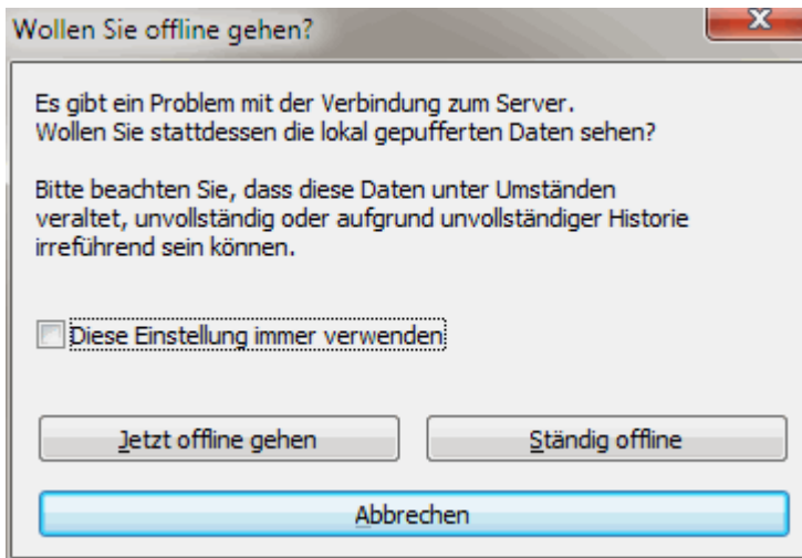
Abbildung 4.28. Offline gehen
