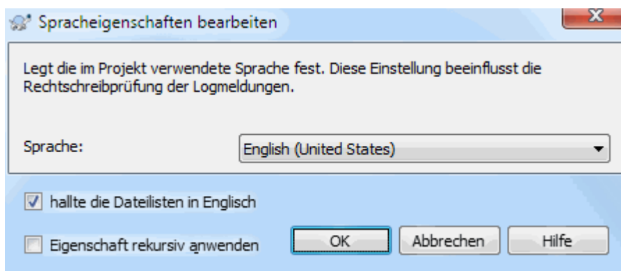
Abbildung 4.46. Sprach-Eigenschaftsseite
