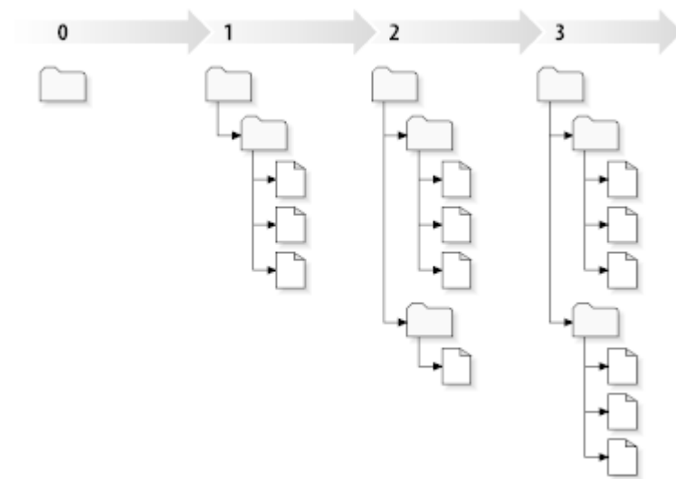
Abbildung 2.7. Das Projektarchiv
