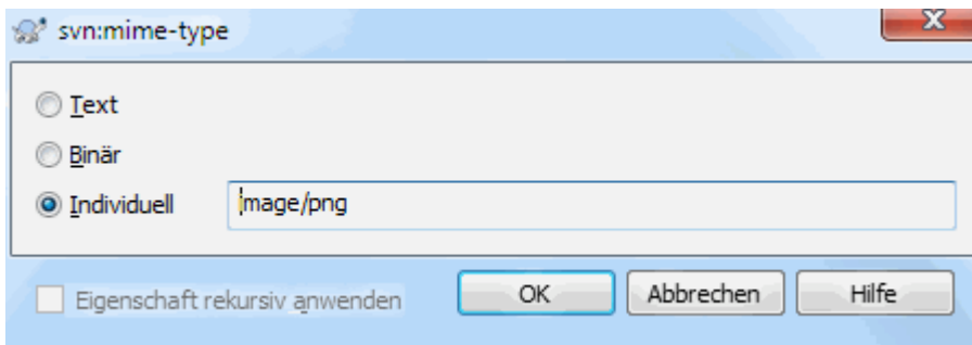
Abbildung 4.47. svn:mime-type Eigenschaftsseite
