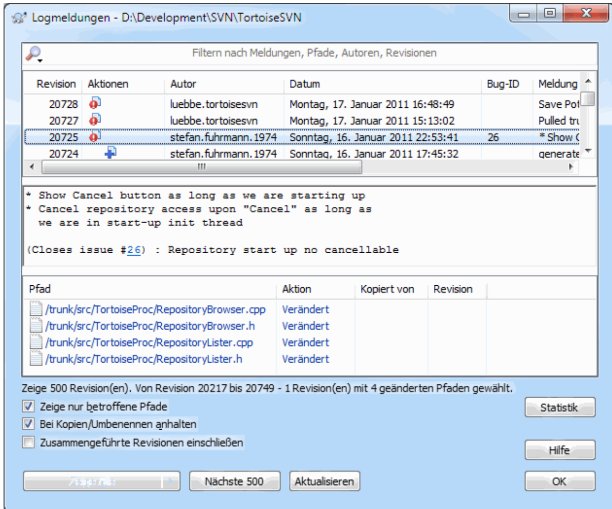
Abbildung 1.4. Der Log-Dialog
