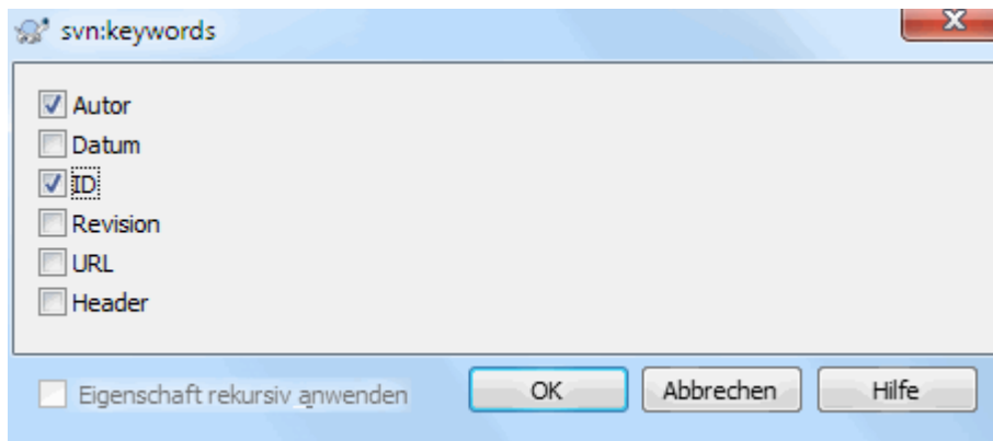
Abbildung 4.42. svn:keywords Eigenschaftsseite
