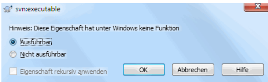
Abbildung 4.49. svn:executable Eigenschaftsseite
