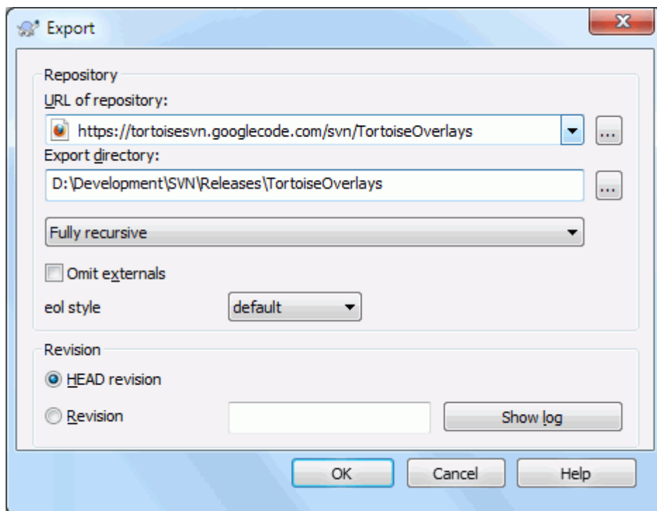
Slika 4.67. Izvoz-iz-URL dijalog
