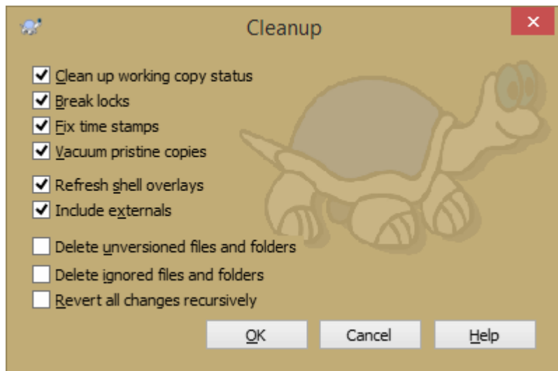
Slika 4.35. Dijalog čišćenja
