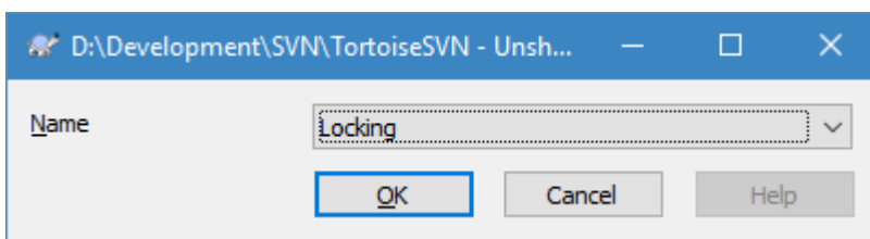
Рисунок 4.17. Unshelve dialog
