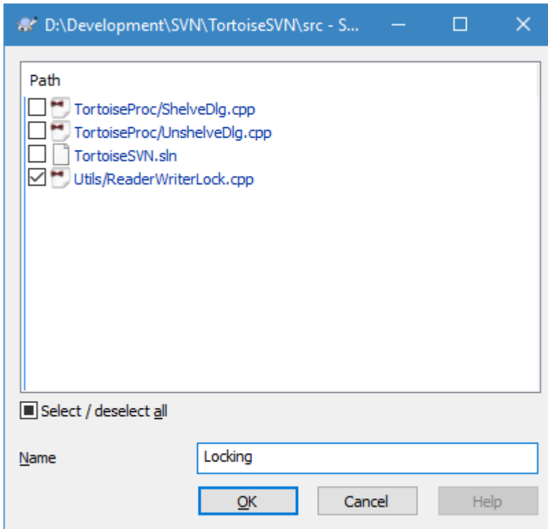
Рисунок 4.16. Shelve dialog
