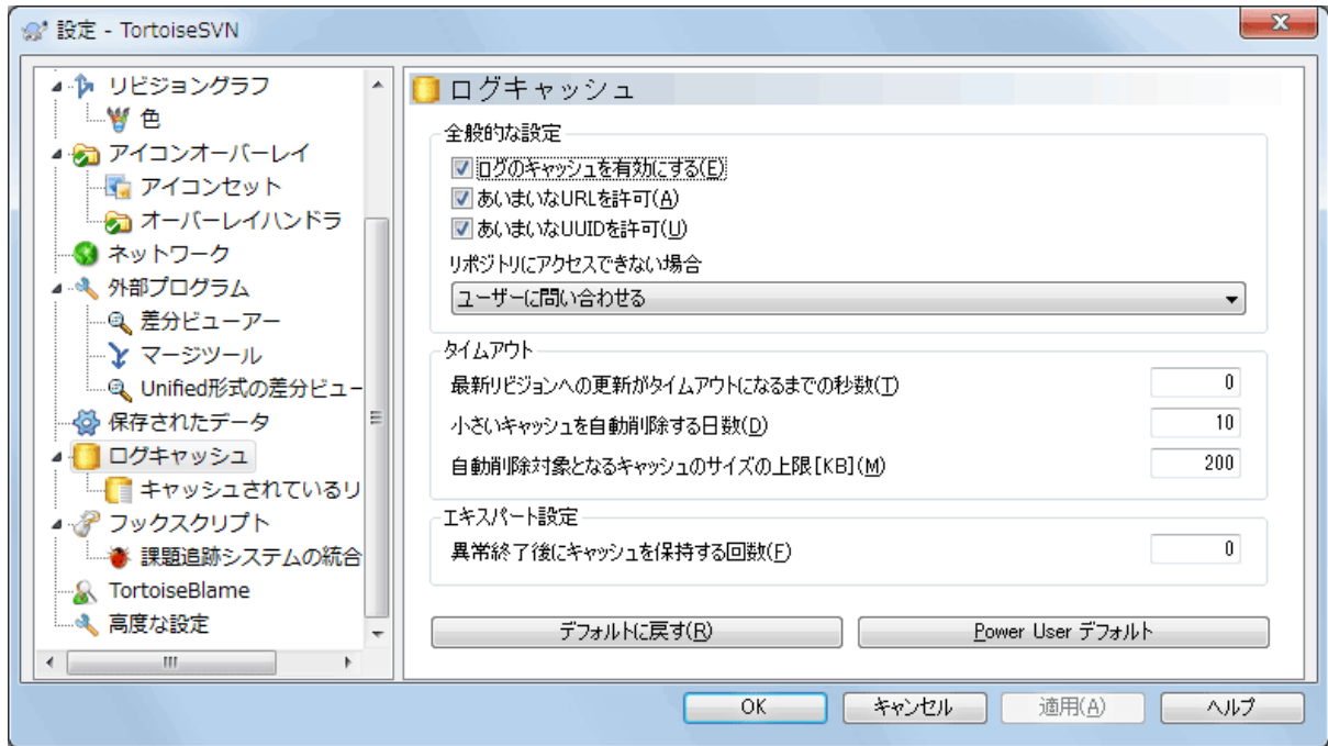
図4.87 設定ダイアログの「ログキャッシュ」ページ
