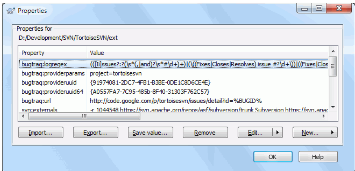
图 4. 34. Subversion 属性页
