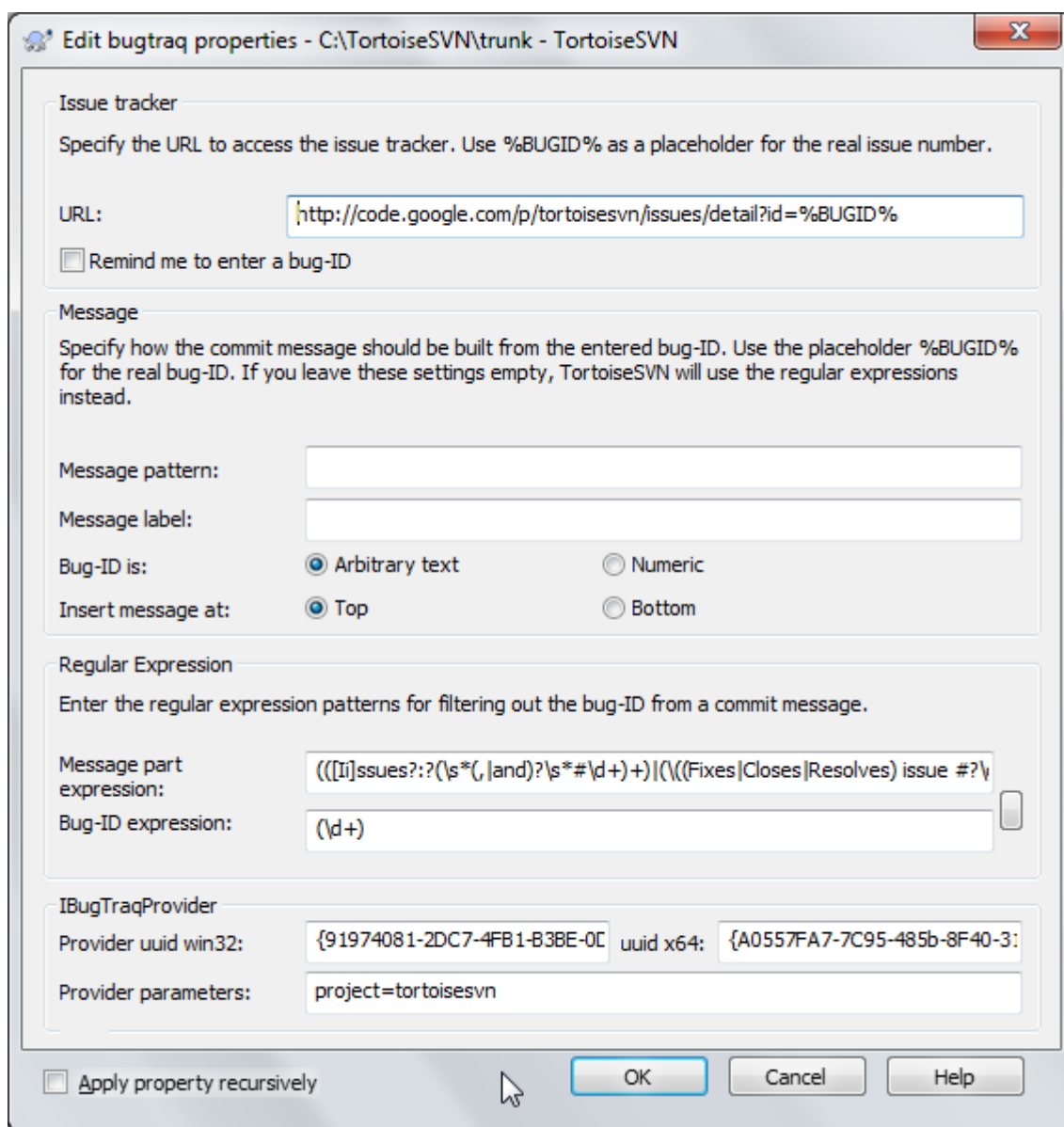
图 4.44. tsvn:bugtraq 属性页
