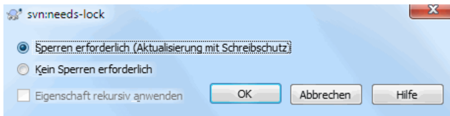
Abbildung 4.46. svn:needs-lock Eigenschaftsseite
