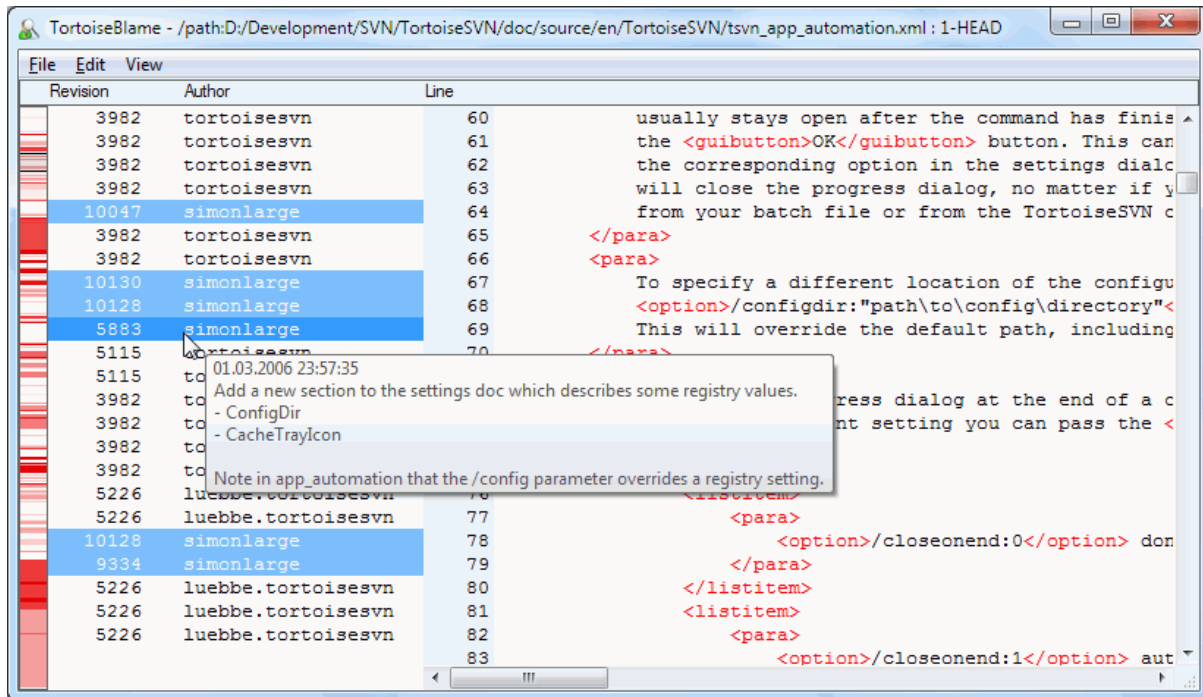
Abbildung 4.59. TortoiseBlame
