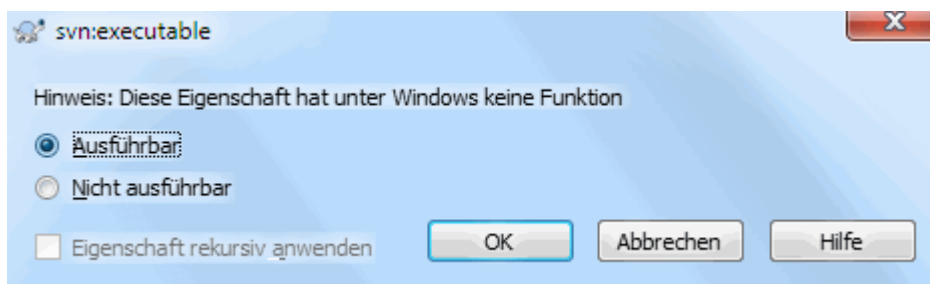
Abbildung 4.47. svn:executable Eigenschaftsseite
