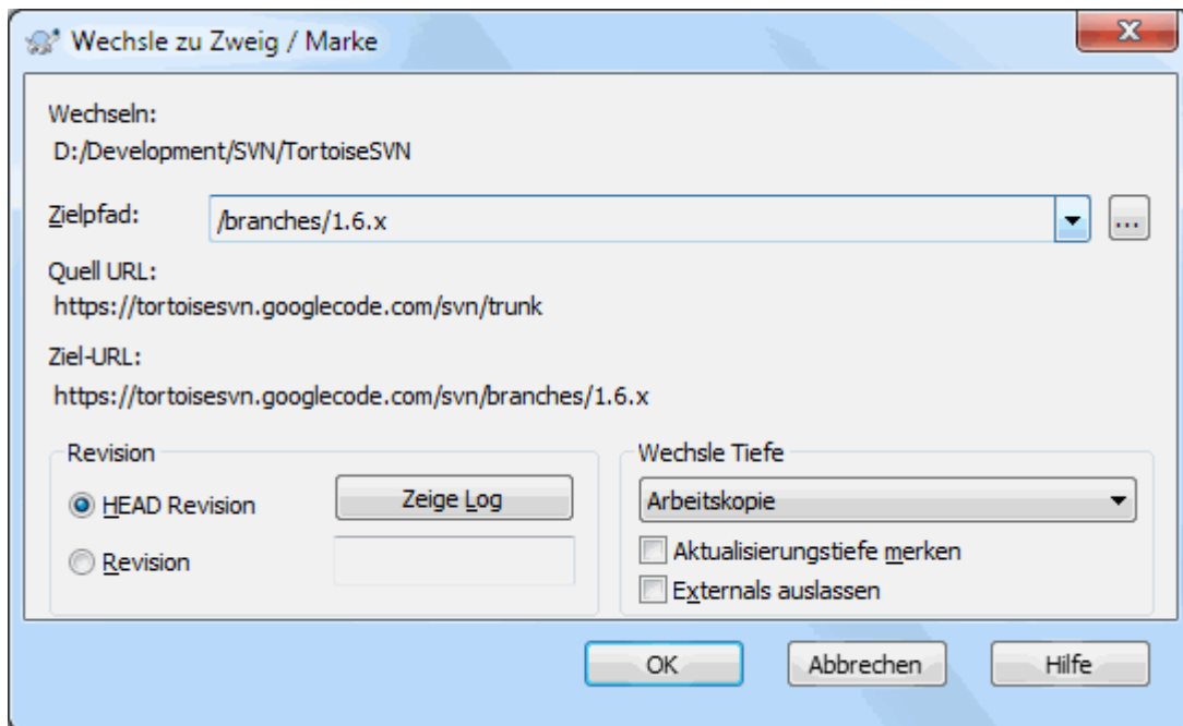
Abbildung 4.50. Der Wechseln-Zu-Dialog
