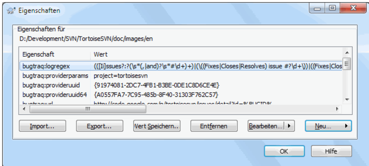
Abbildung 4.35. Subversion Eigenschaftsseite
