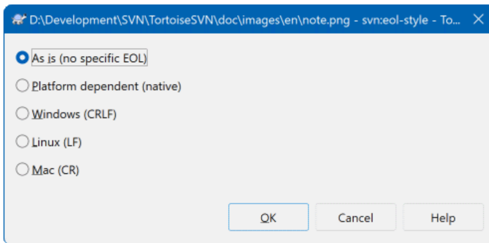
图 4.44. svn:eol-style 属性页
