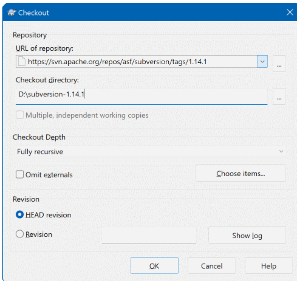
图 4.7. 检出对话框
