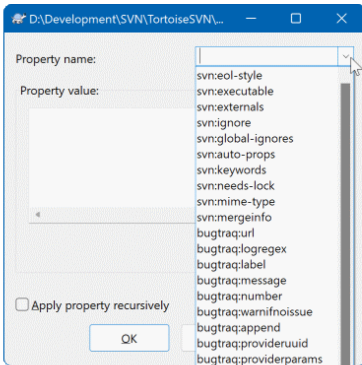
图 4.36. 增加属性
