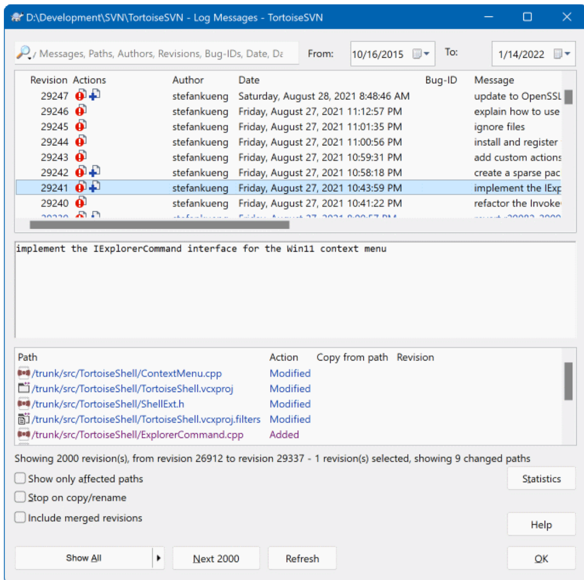
Gambar 4.18. Dialog Log Revisi
