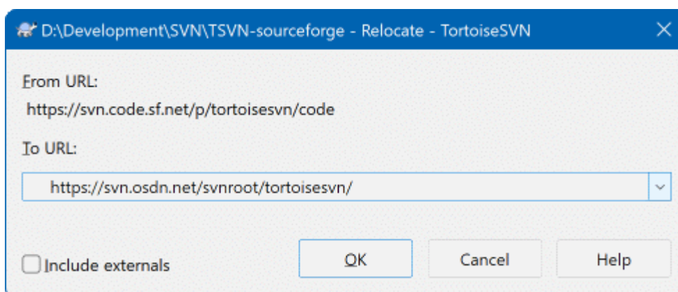
Gambar 4.69. Dialog Relokasi
