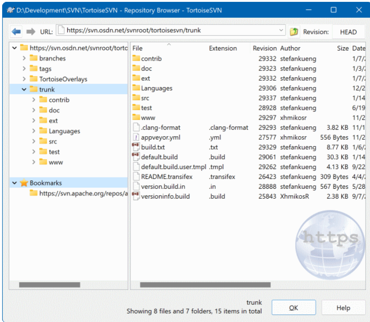
Gambar 4.66. Browser Repositori
