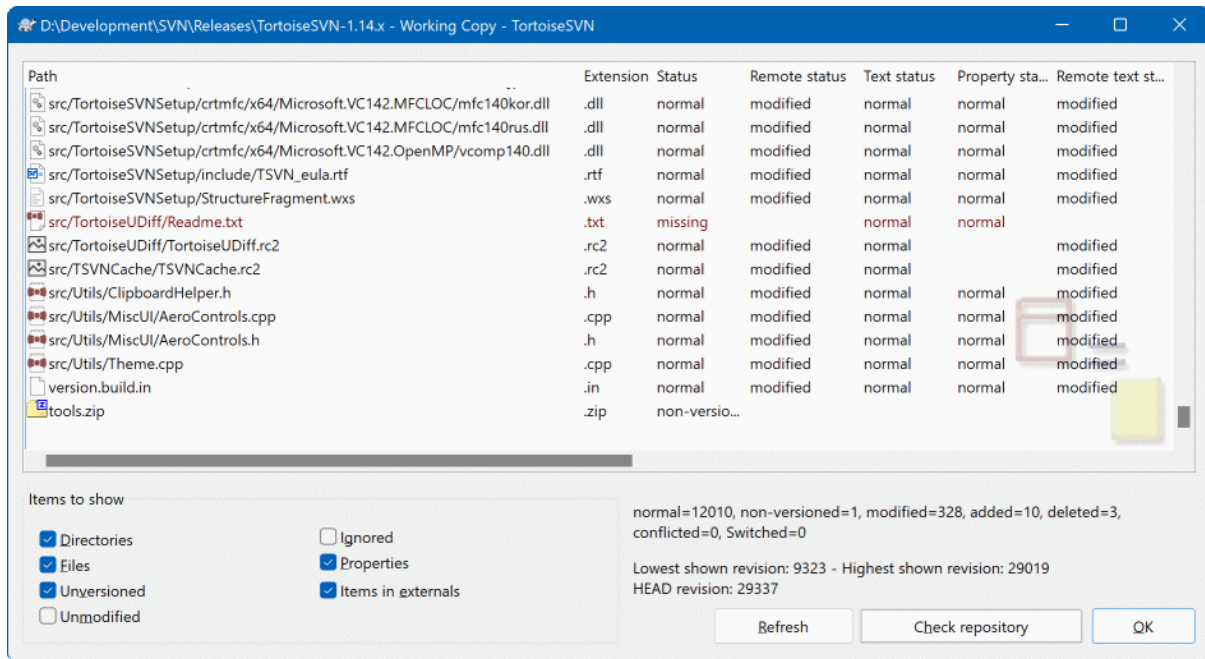
Gambar 4.14. Periksa Modifikasi
