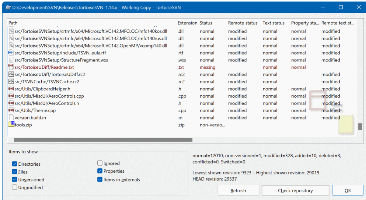
Gambar 4.62. Dialog Pemeriksaan Modifikasi
