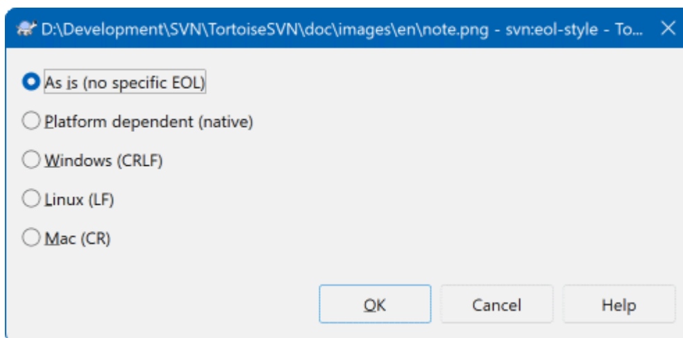
Gambar 4.46. svn:eol-style property page
