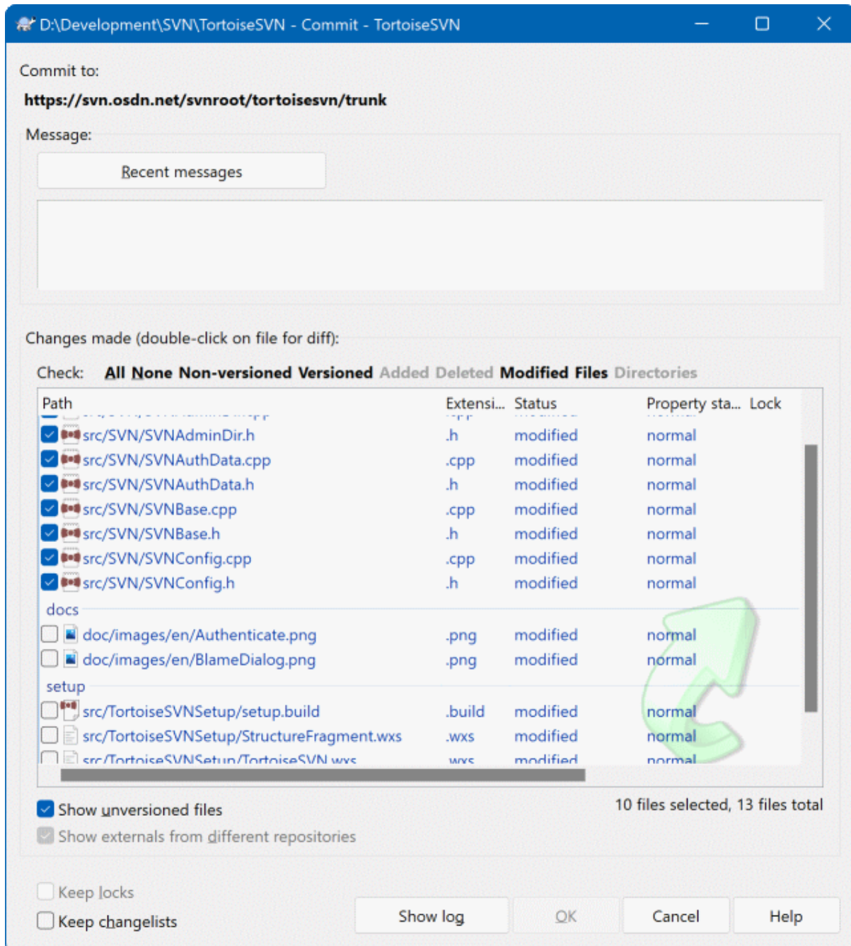
Gambar 4.15. Dialog Komit dengan Daftar Perubahan
