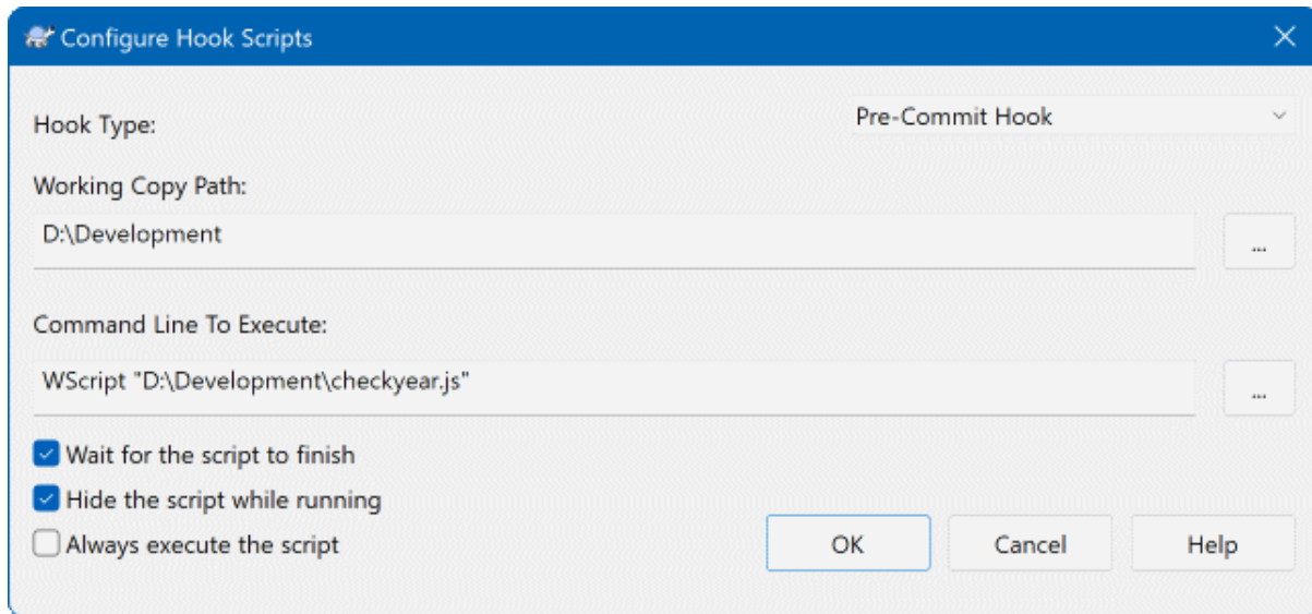
Gambar 4.90. Dialog Seting, Konfigurasi Naskah Hook
