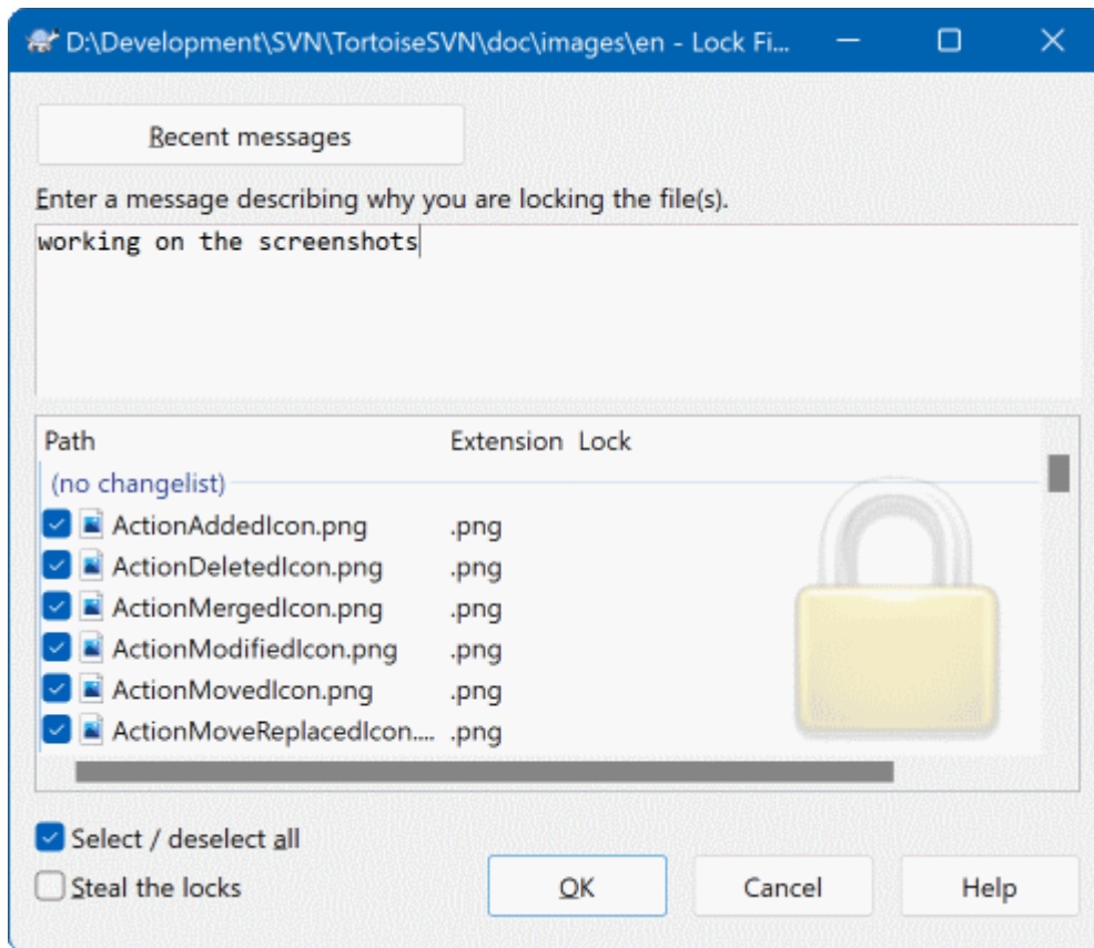
Gambar 4.61. Dialog Penguncian
