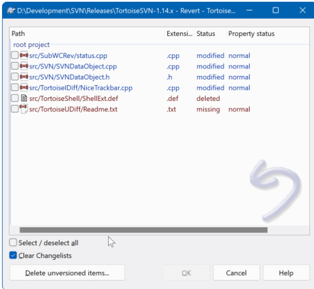
Gambar 4.35. Dialog Pulihkan
