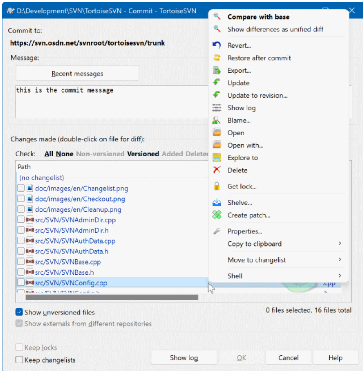
Gambar 4.8. Dialog Komit
