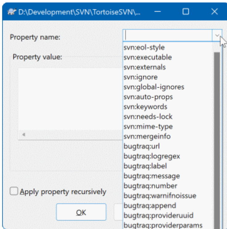
Gambar 4.38. Menambah properti
