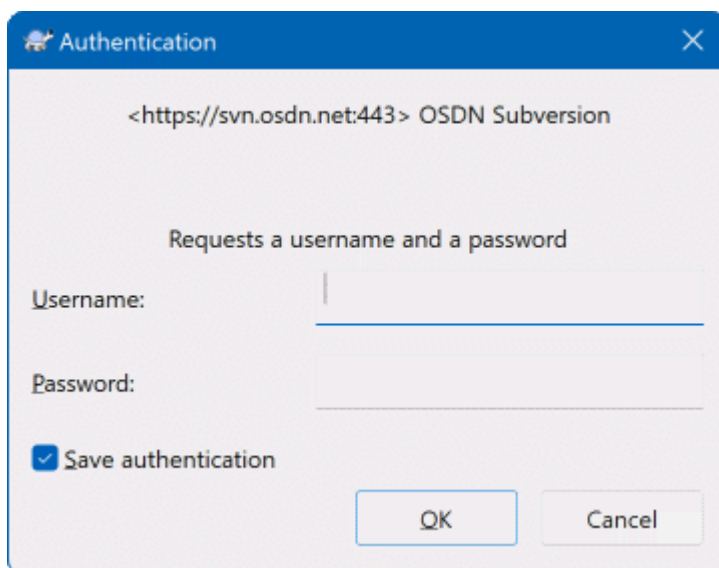
Gambar 4.5. Dialog Otentikasi
