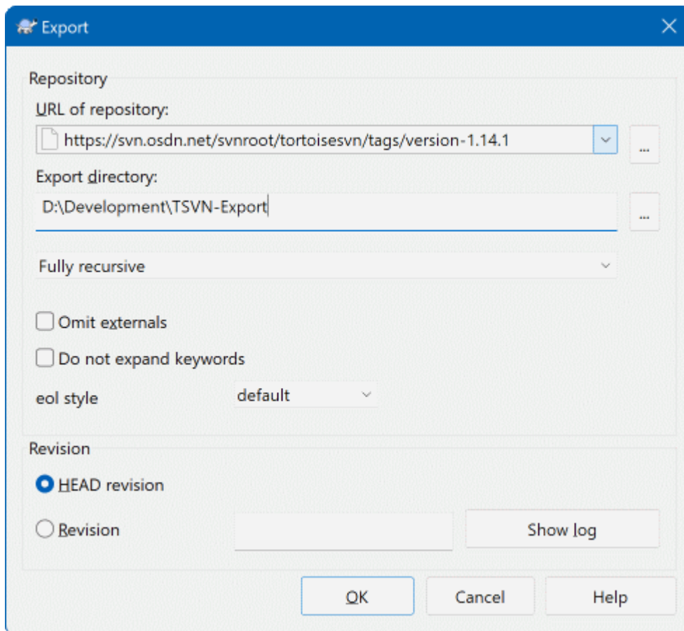
Gambar 4.68. Dialog Ekspor-dari-URL
