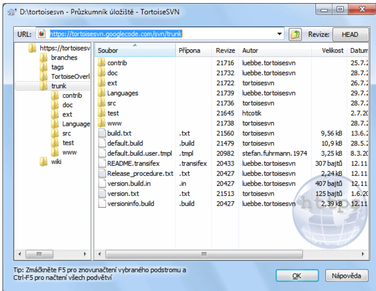
Obrázek 4.66. Průzkumník Úložiště
