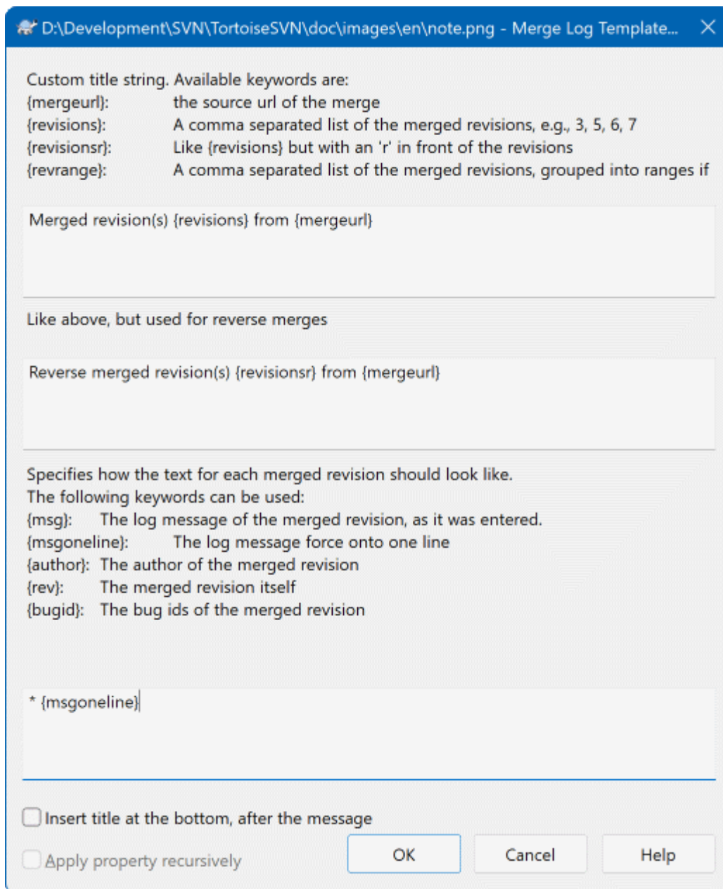
図4.53 プロパティダイアログのマージログメッセージのテンプレート設定
