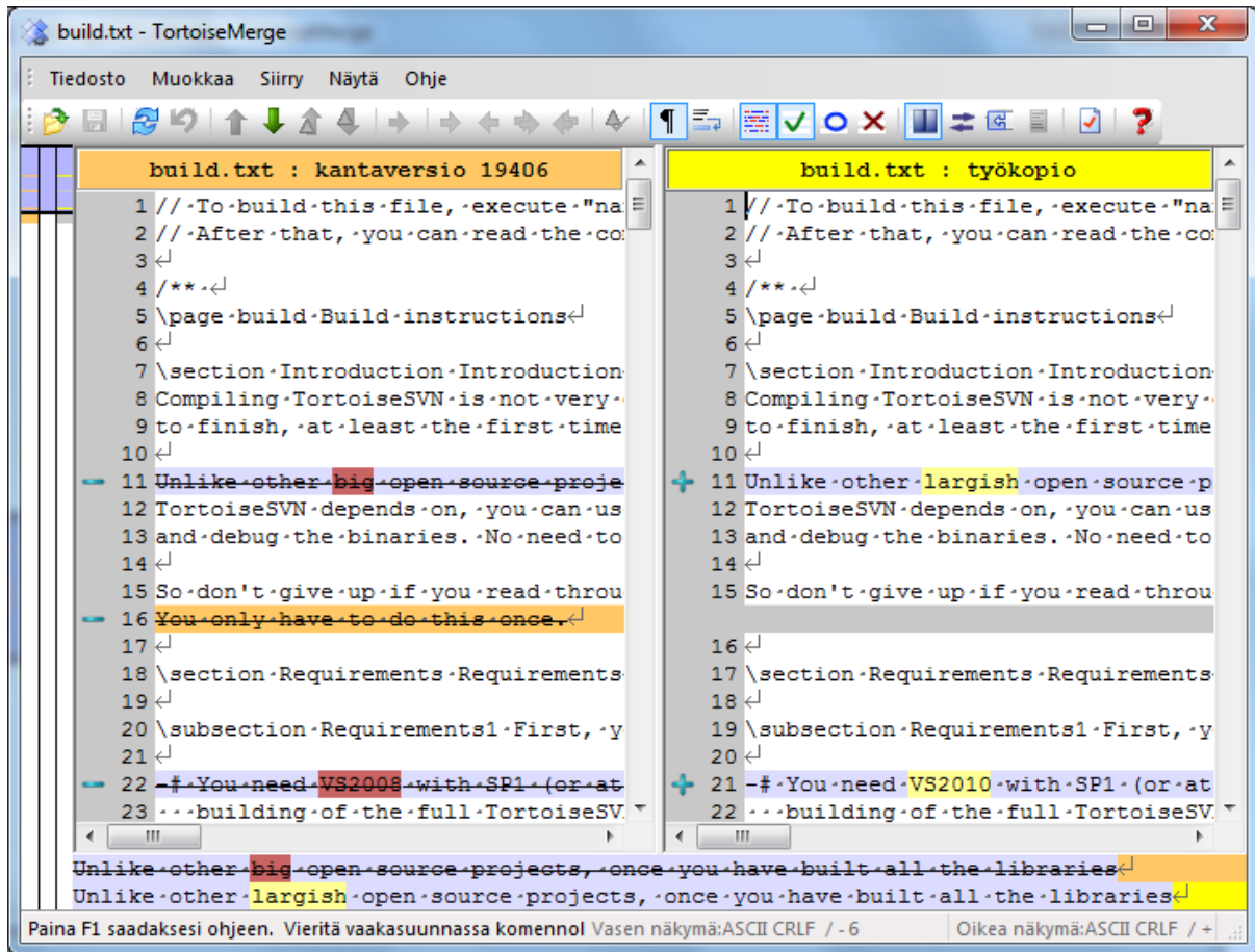
Kuva 1.3. Tiedostojen vertaileminen
