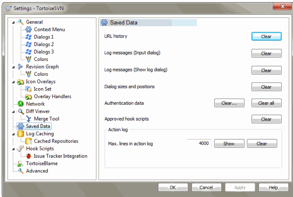
Obrázok 4.82. Dialógové okno Nastavenia, stránka Uložené údaje
