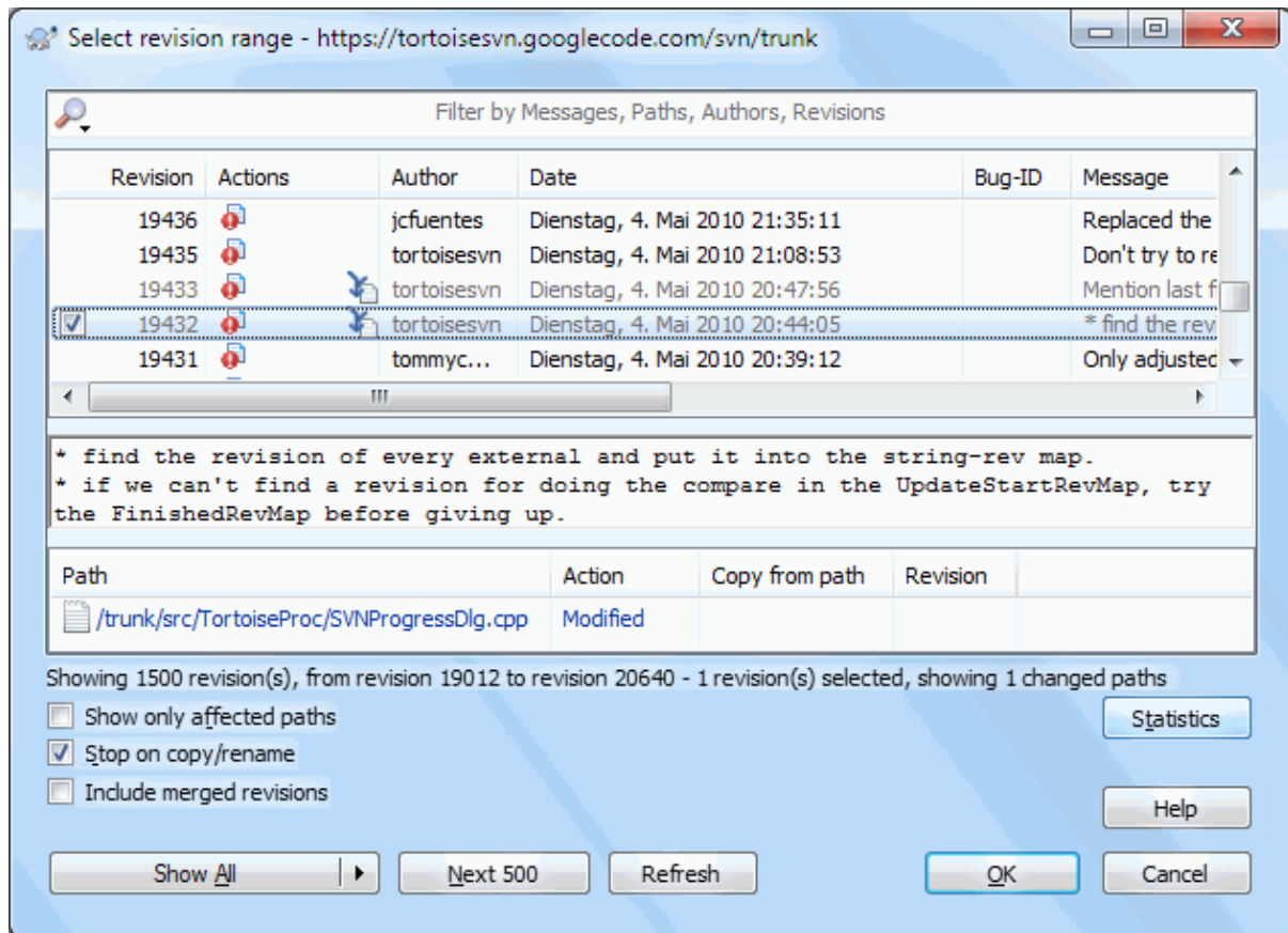
Obrázok 4.24. Dialógové okno záznamu zobrazujúce revízie sledovania zlúčenja
