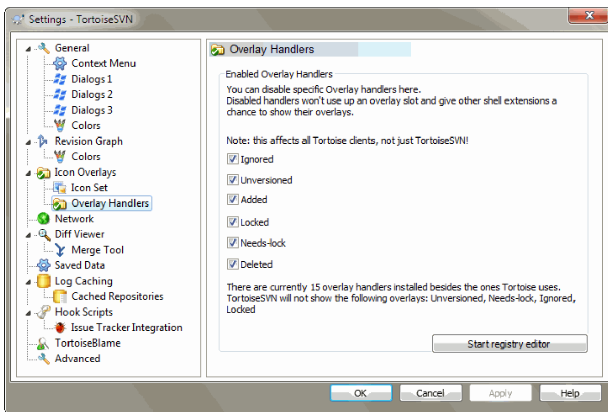
Obrázok 4.78. Dialógové okno Nastavenia, stránka Manipulátory ikon
