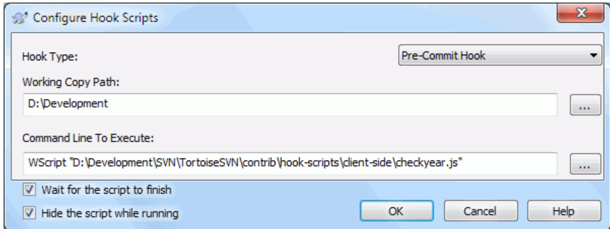
Obrázok 4.86. Dialógové okno Nastavenia, Konfigurácia skriptov háku
