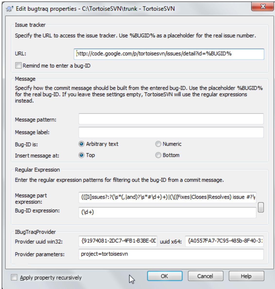
Obrázok 4.66. Dialógové okno Vlastností Bugtraq (sledovania chýb)
