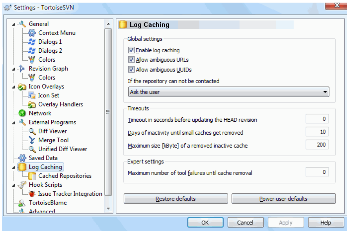
Obrázok 4.83. Dialógové okno Nastavenia, stránka Uchovanie záznamov
