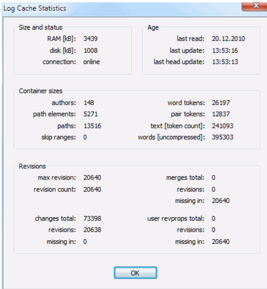
Obrázok 4.84. Dialógové okno Nastavenia, Štatistika zásobníka záznamu
