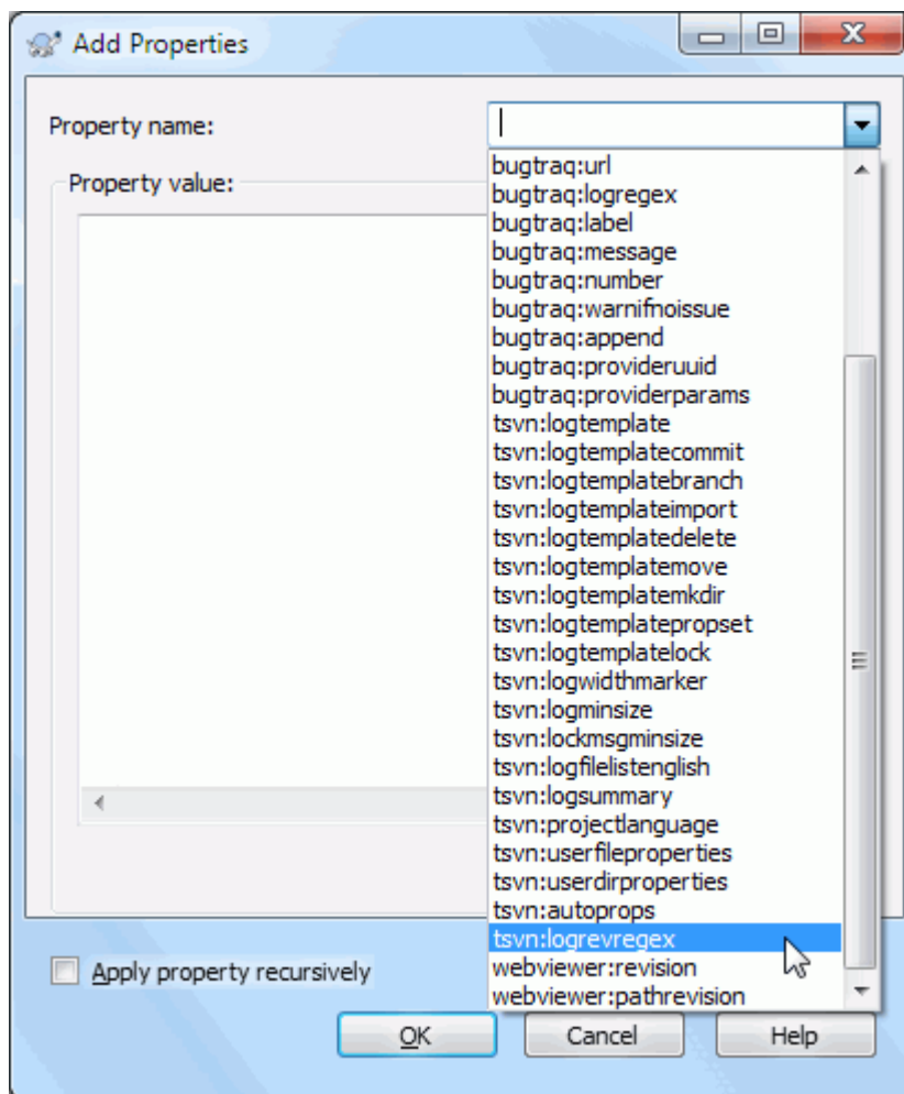
Obrázok 4.38. Pridávanie vlastností
