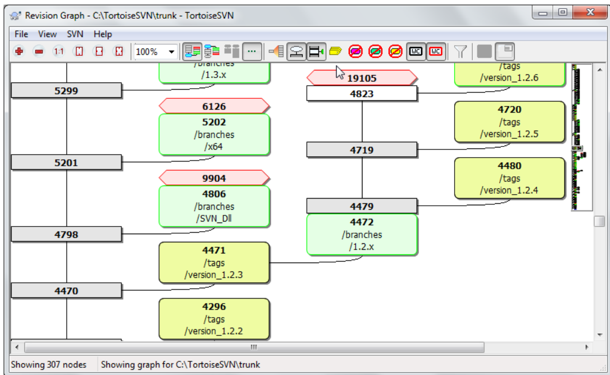
Obrázok 4.63. Graf revízií
