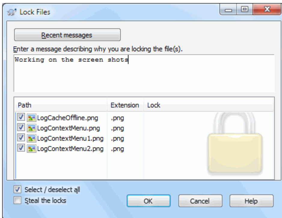
Obrázok 4.57. Dialóg Zamykanie
