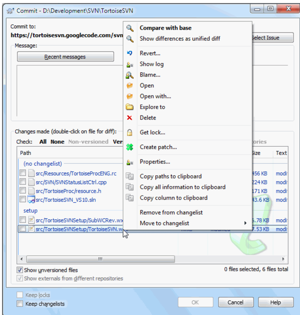
Obrázok 4.8. Dialóg odovzdania
