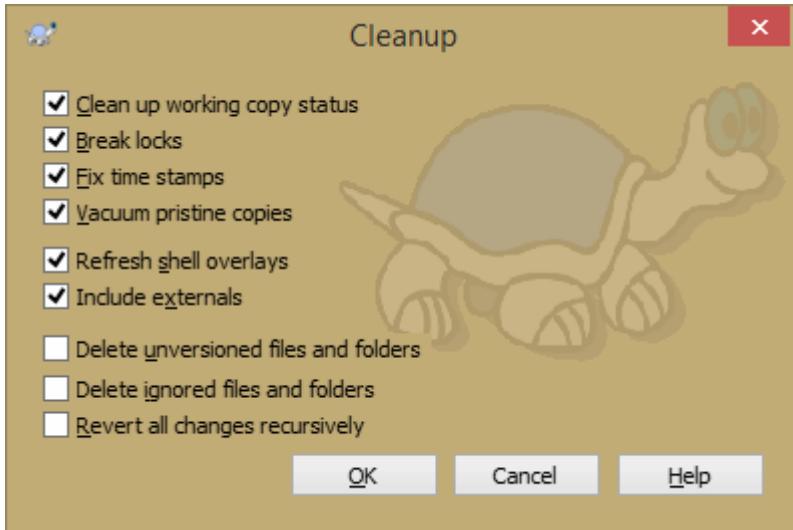
Obrázok 4.36. Dialóg Vyčistiť
