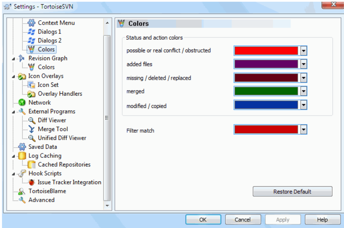
Obrázok 4.73. Dialógové okno Nastavenia, stránka Farby
