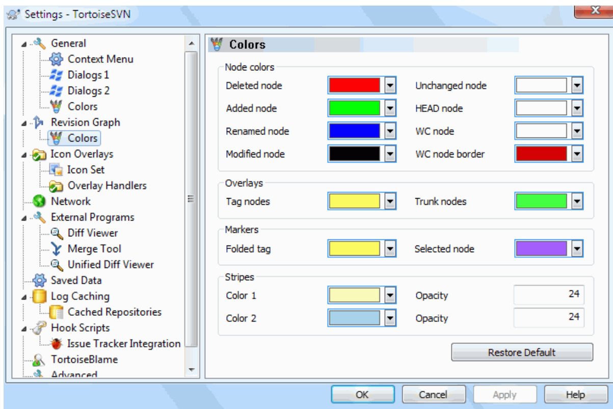
Obrázok 4.75. Dialógové okno Nastavenia, stránka Farby grafu revízií
