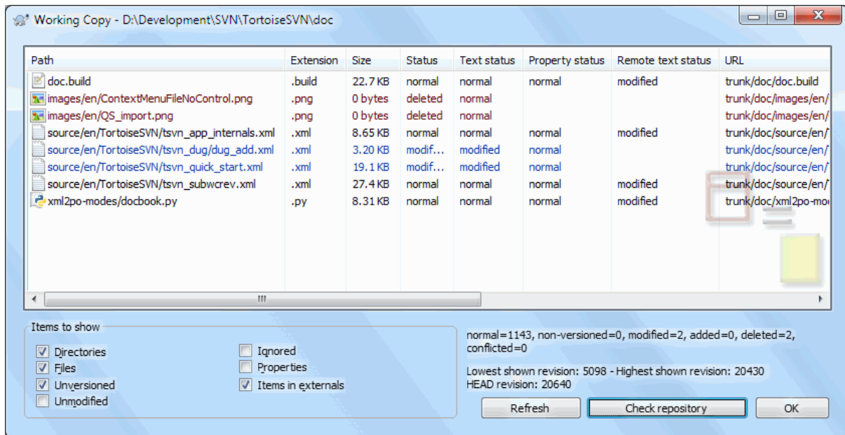
Obrázok 4.14. Skontrolovať zmeny
