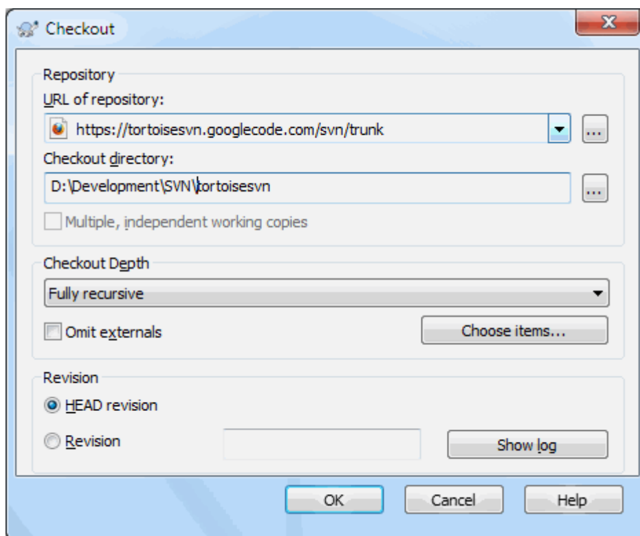
Obrázok 4.7. Dialóg overenia
