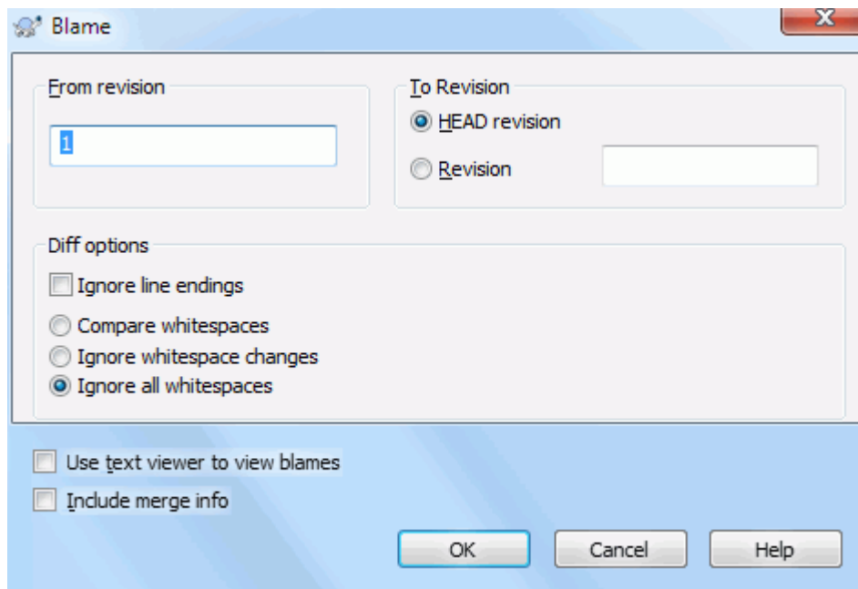
Obrázok 4.60. Dialóg poznámky/zdpovednosti
