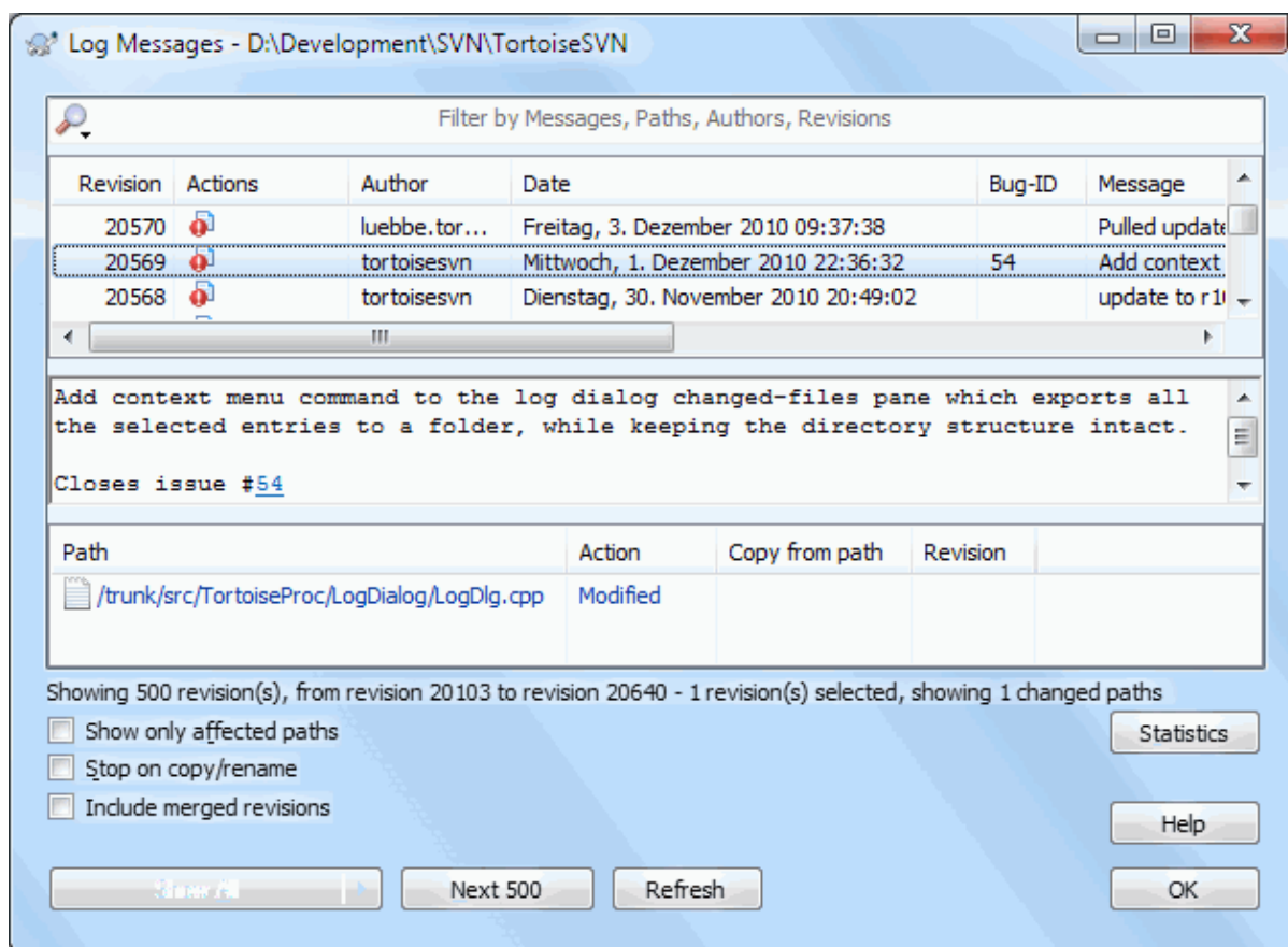
Obrázok 1.4. Dialóg záznamu
