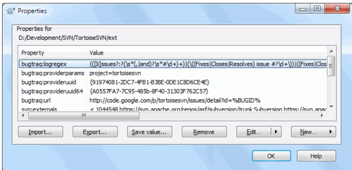
Obrázok 4.37. Stránka vlastností Subversion
