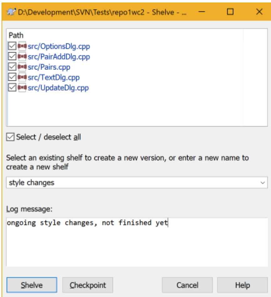
图 4.16. Shelve dialog
