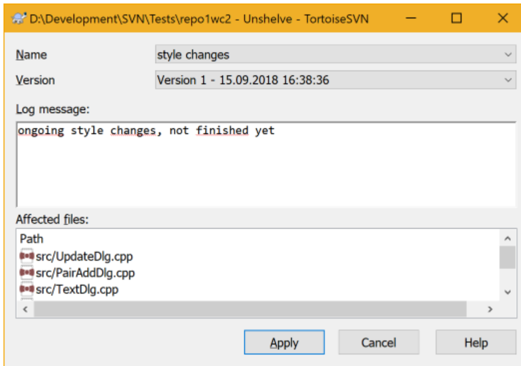
图 4.17. Unshelve dialog
